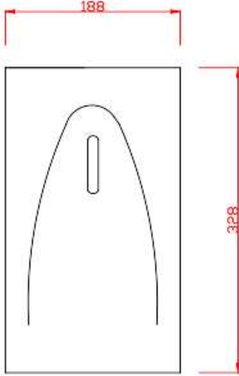
ÖN GÖRÜNÜŞ
