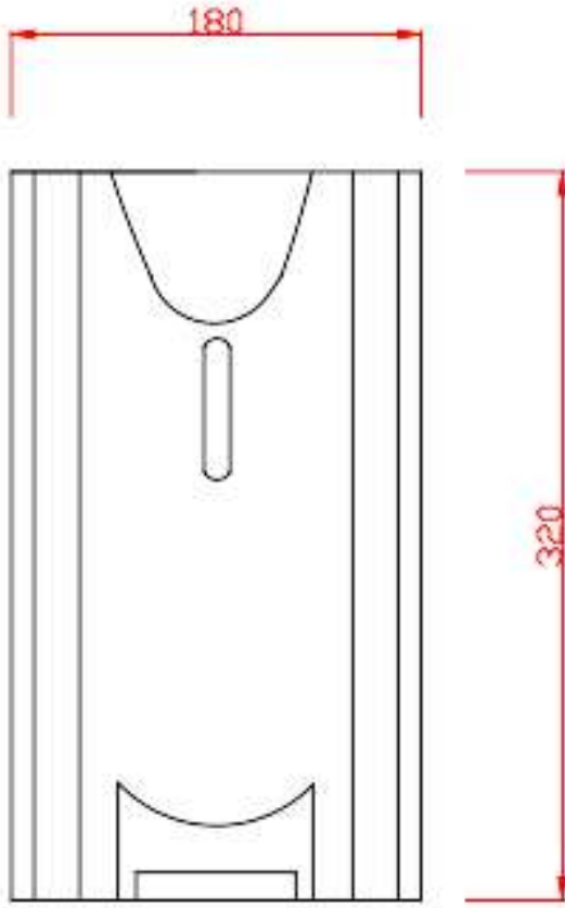
ÖN GÖRÜNÜŞ
