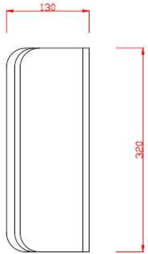
YAN GÖRÜNÜŞ
