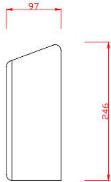
YAN GÖRÜNÜŞ
