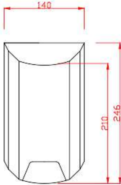
ÖN GÖRÜNÜŞ
